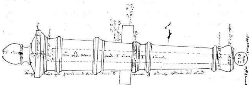
Чертеж 3-х фунтовой пушки, по которому отливали пушки на Каменском заводе
